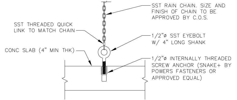
13 RAIN CHAIN BOTTOM CONNECTION N.T.S.
