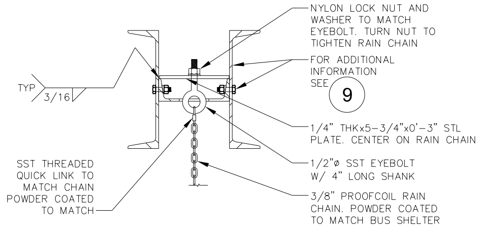
12 RAIN CHAIN TOP CONNECTION N.T.S.
