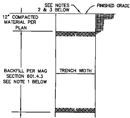
TYPE 'B' BACKFILL
