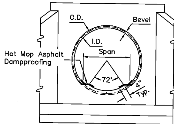
ELEVATION A-A
